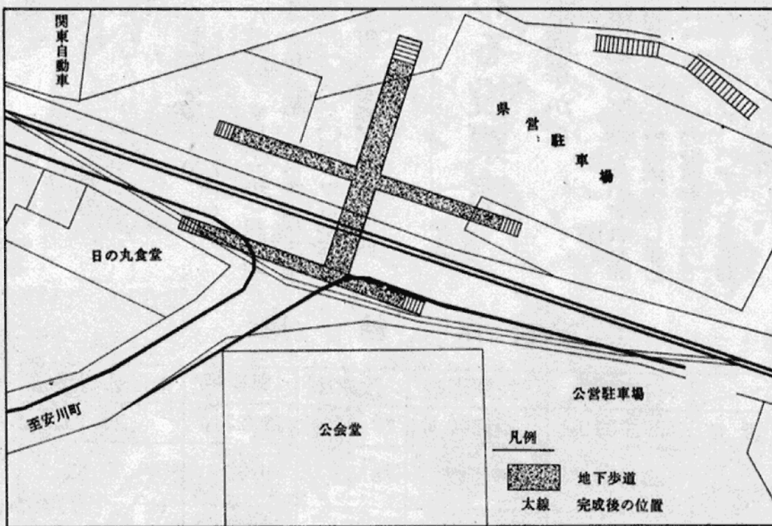
地下横断歩道の建設位置図
