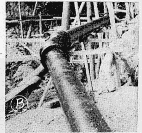
写真B 新しい鉄管を高くあげて臨時に送水管を建設中
